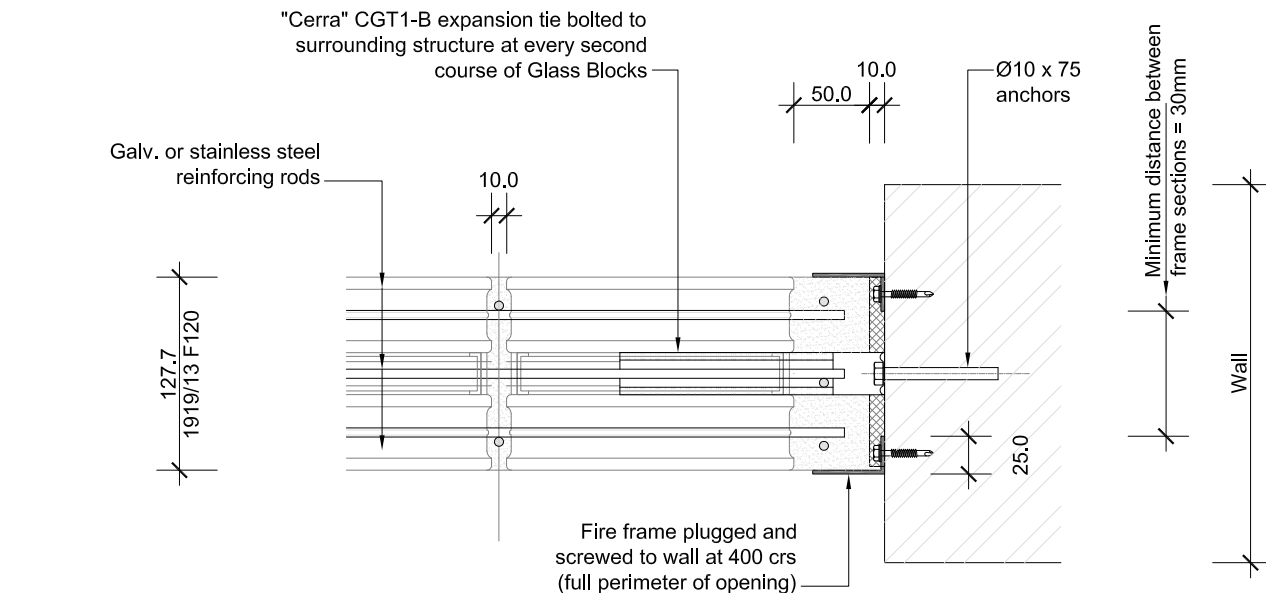
PLAN - JAMB 1:5
