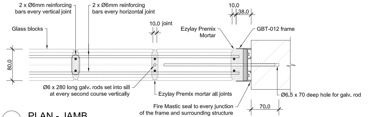
PLAN - JAMB 1:5
